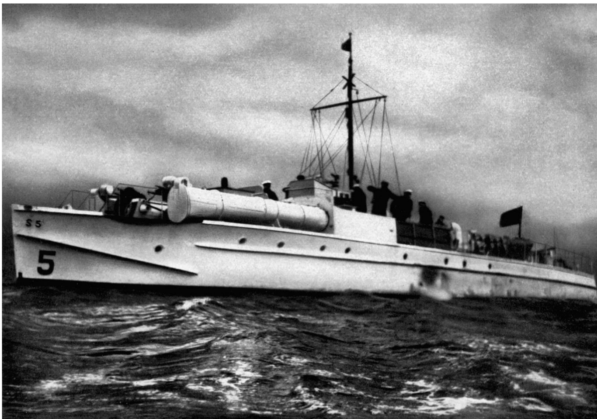
„Хрътките“ на Балтийско море: германски торпеден катер
